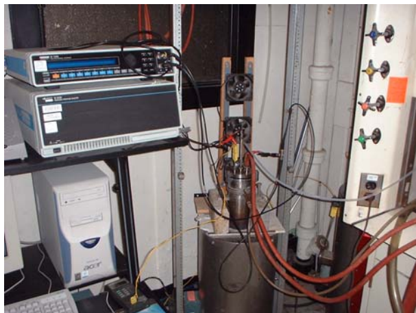
写真3 チタンの新製造プロセス研究のための予備的な実験装置
